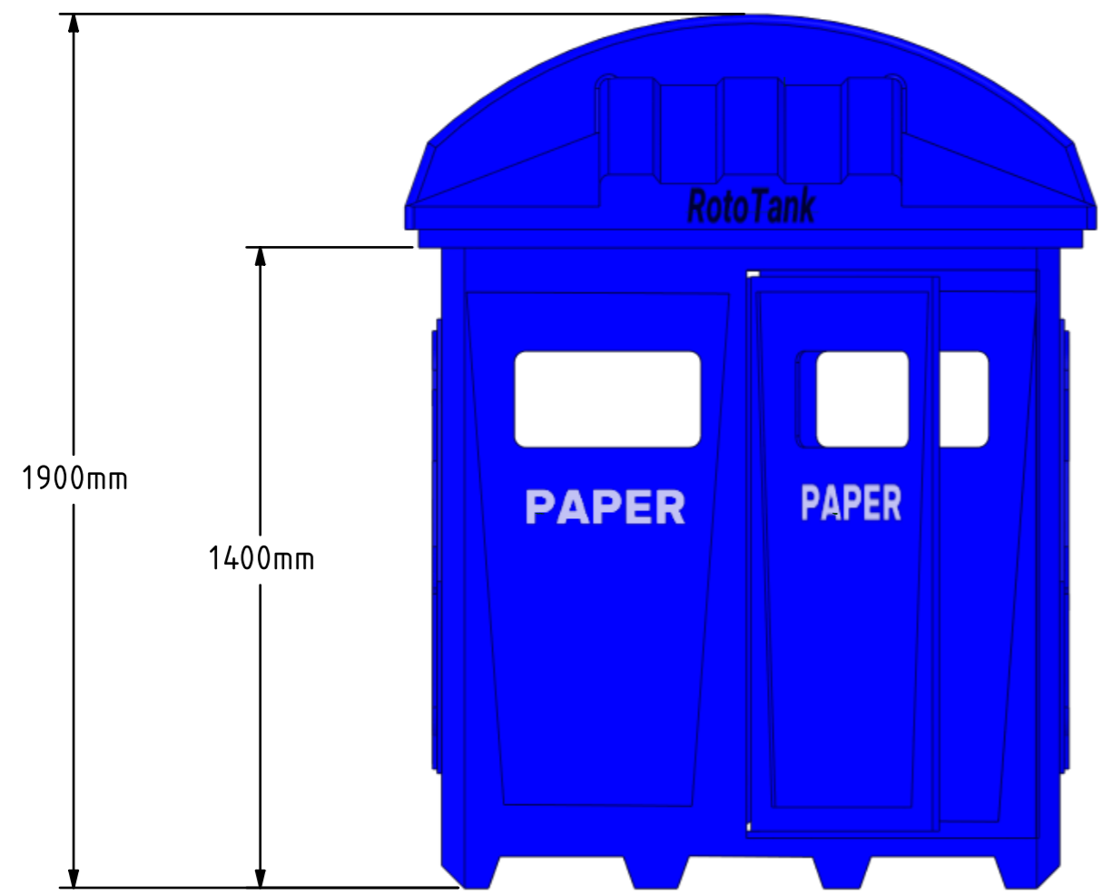
SCALE 1:15
