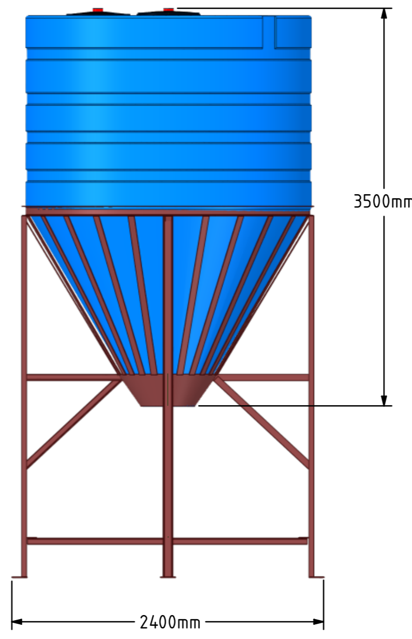
SCALE 1:30
